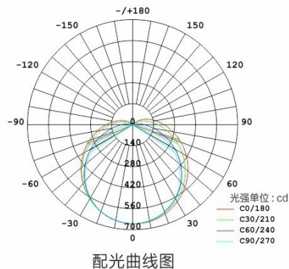
配光曲线图
