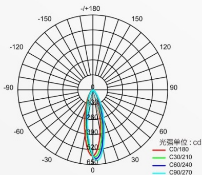
配光曲线图
