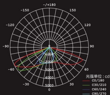
配光曲线图
