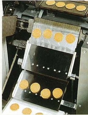
■スクレイパー装置 Scraper Device
